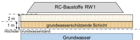
Abb. 29: Eingeschränkter offener Einbau (RW1) 24 [Mettke]
